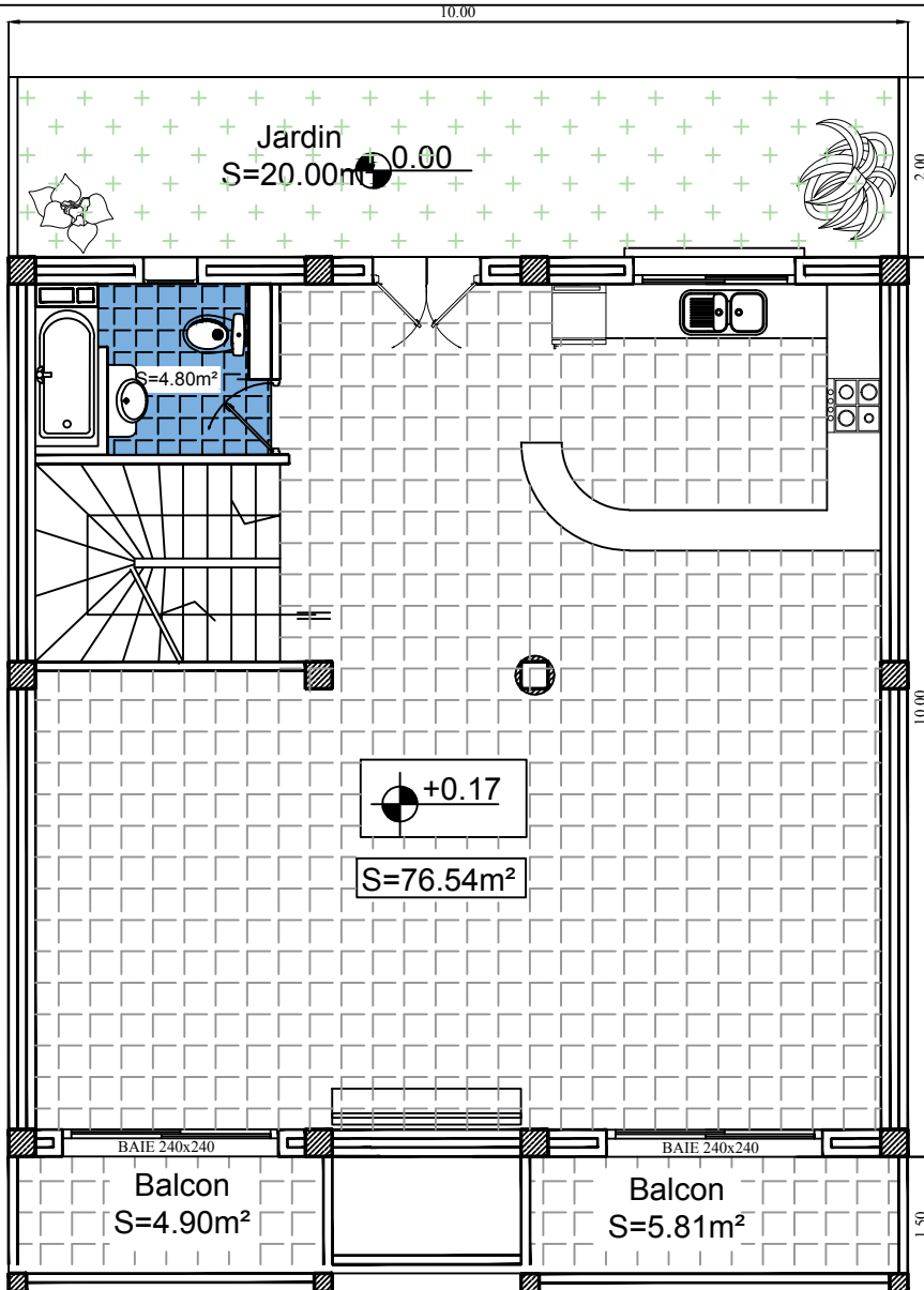
PLAN RDC
