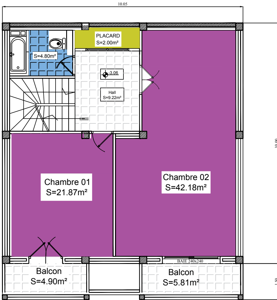
PLAN ENTRE SOL 01
